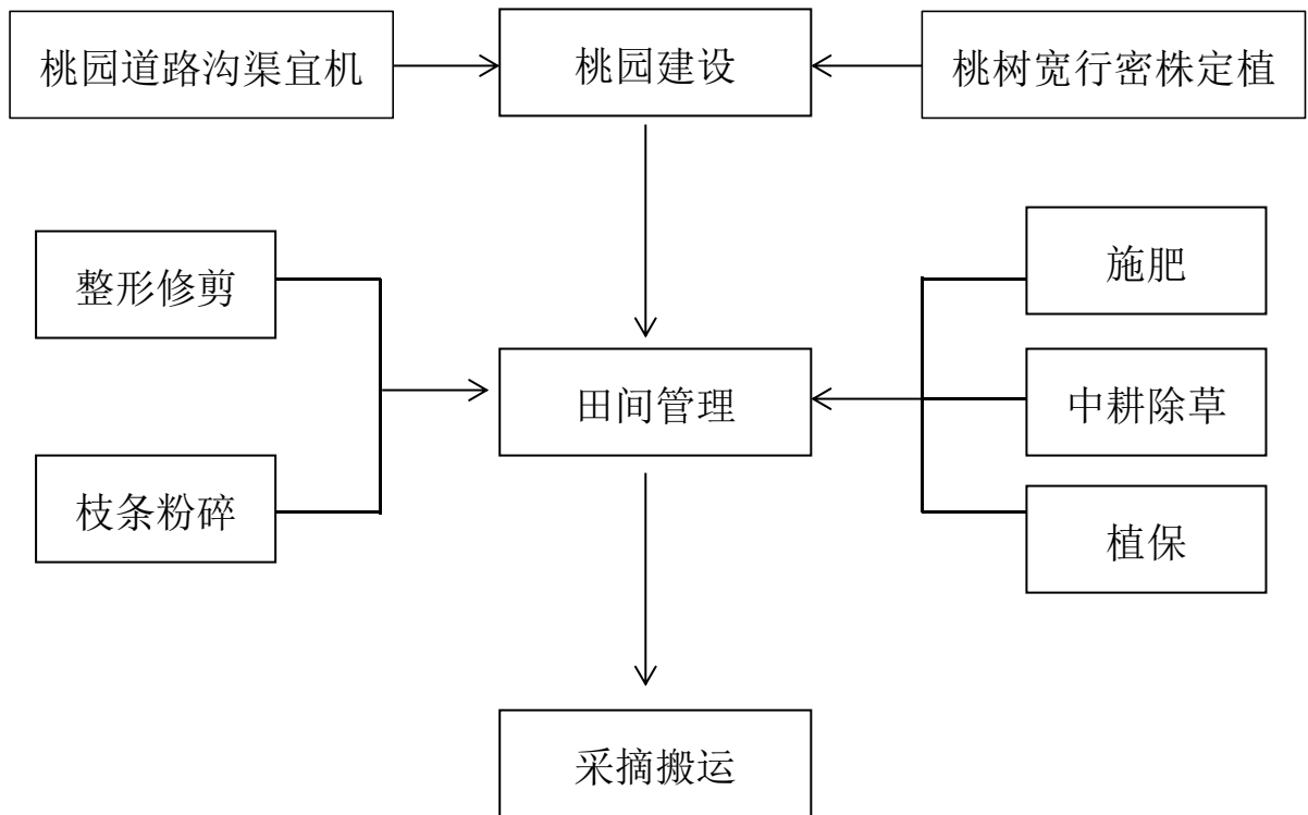
图 B.1 桃树全程机械化生产技术路线图
